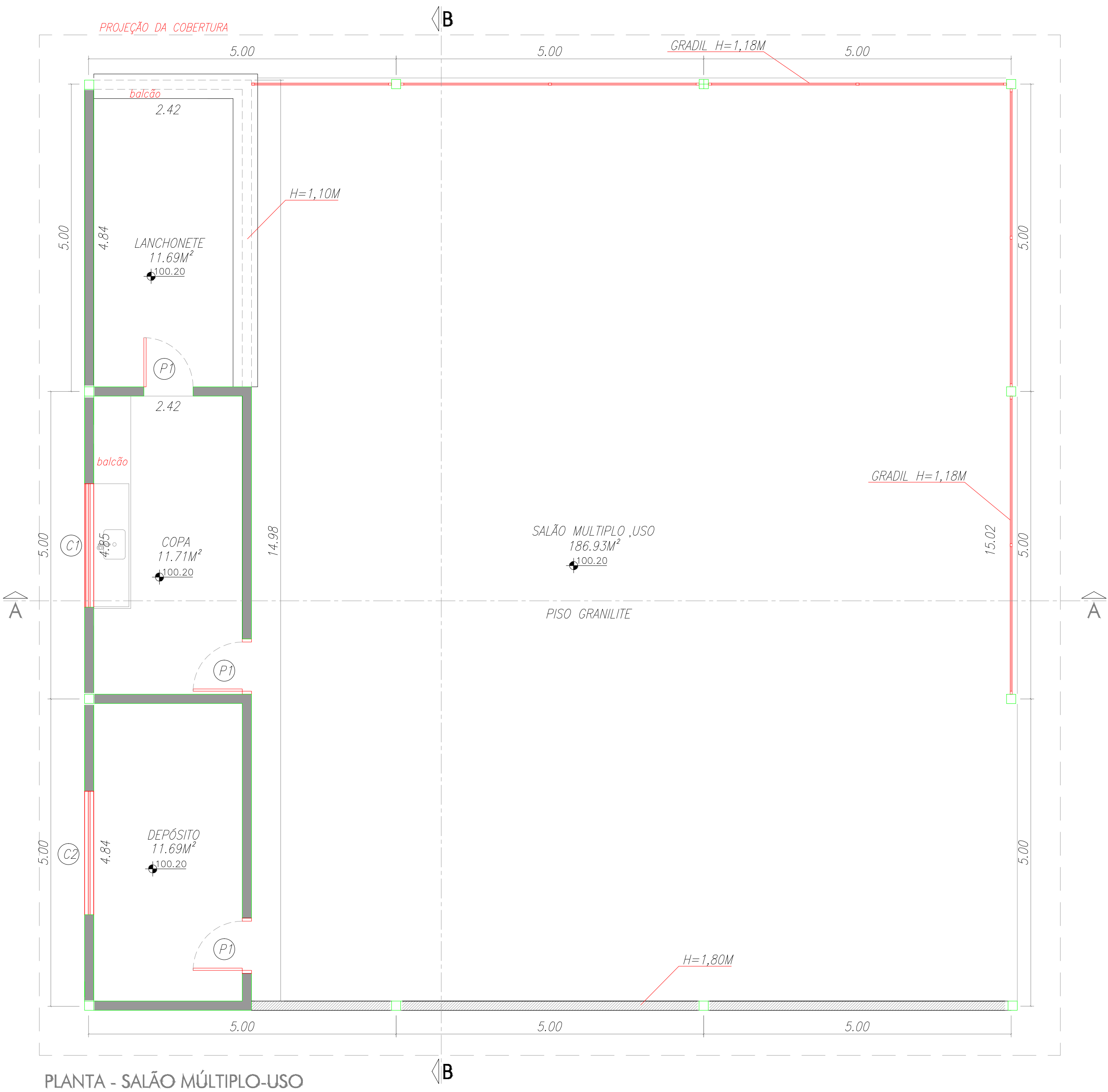
PLANTA - SALÃO MÚLTIPLO-USO
