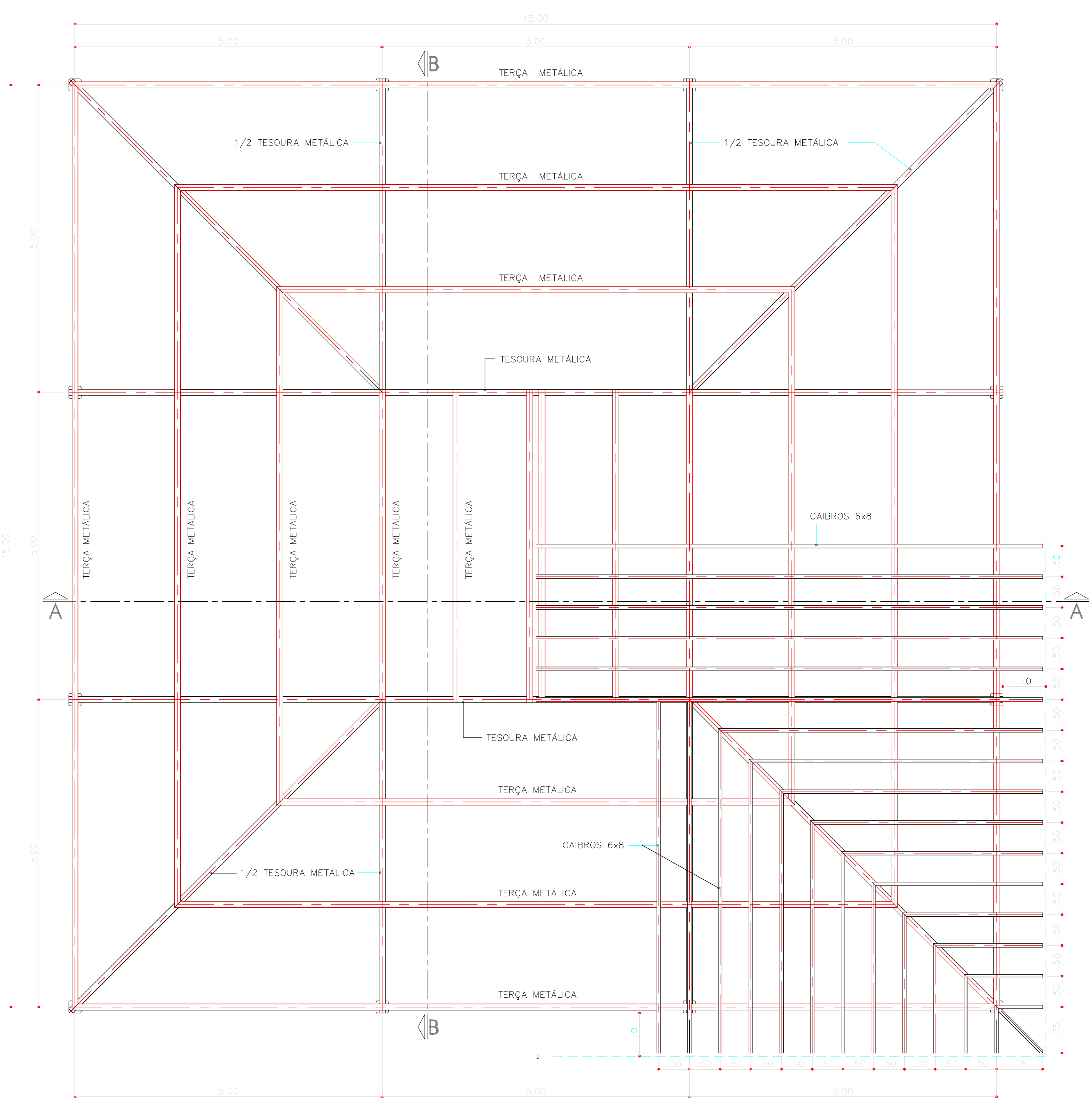
PLANTA - ESTRUTURA DO TELHADO
